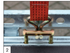
Serienausstattung: TÜV-geprüfte Verzurrbügel, integriert im Seitenrahmen: 1000 daN das Stück.
