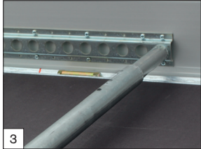
Option: Radstopper Modell „Combi Protect Rail“.
